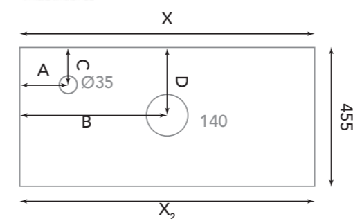
Encimera con agujero para lavabo y grifo
